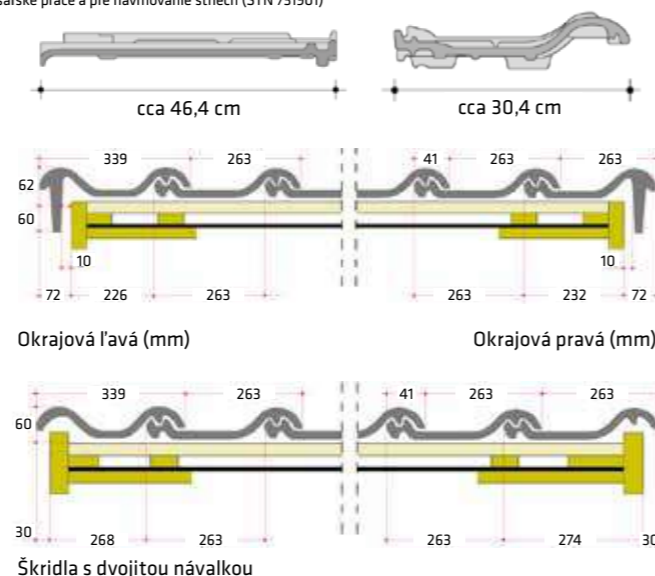
Škridla s dvojitou návalkou
